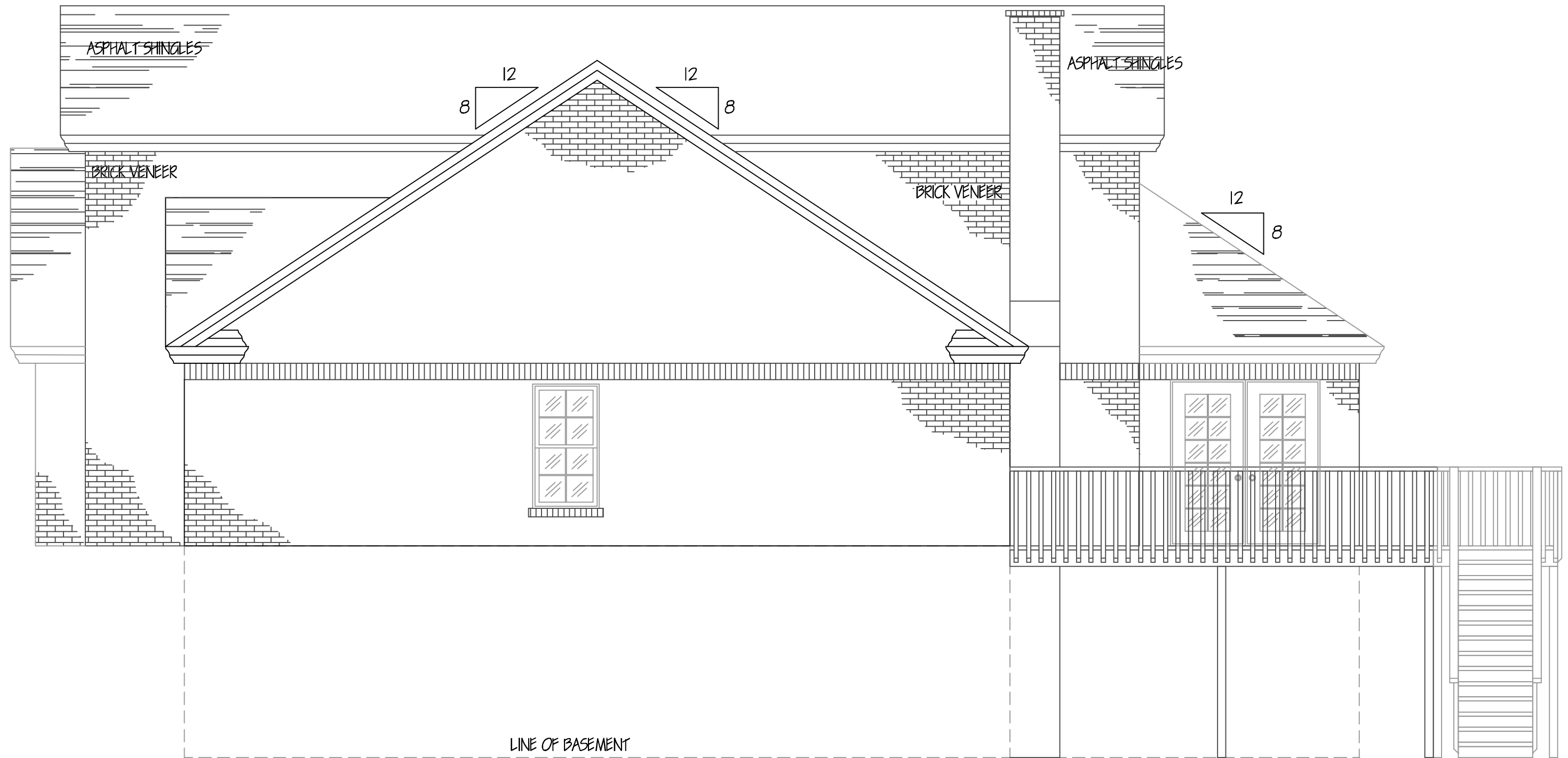
RIGHT ELEVATION
